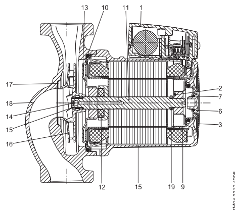
Рис. 33 Насос UPS, модели UPS xx-100
